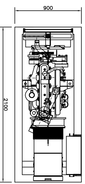
VISTA DALL'ALTO OVER VIEW
